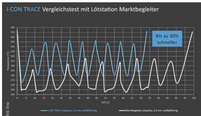
Lötperformance im Vergleich – die i-CON Trace ist bis zu 30 % schneller
